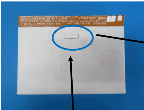
③ ②と反対側の面にこのような形にカッターナイフで切り込みを入れる
